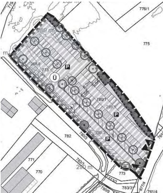
Abb. 1: Ausschnitt Entwurf, Bebauungsplan „Parkplatz Kohlfurtweg“ Stand: 30.01.2023
